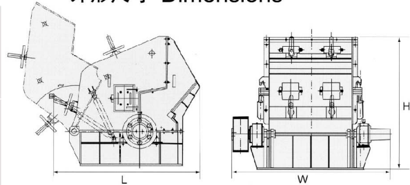
外形尺寸 Dimensions
