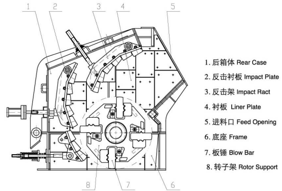
结构图 Structure Drawing
